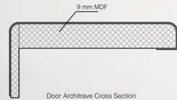
Door Architrave Cross Section
